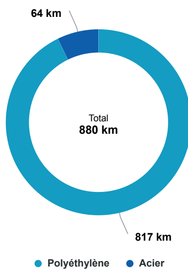
Évolution des canalisations par matière
